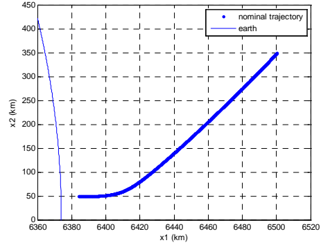
Fig. 1 Nominal trajectory
